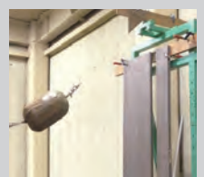
Tes Ketahanan
